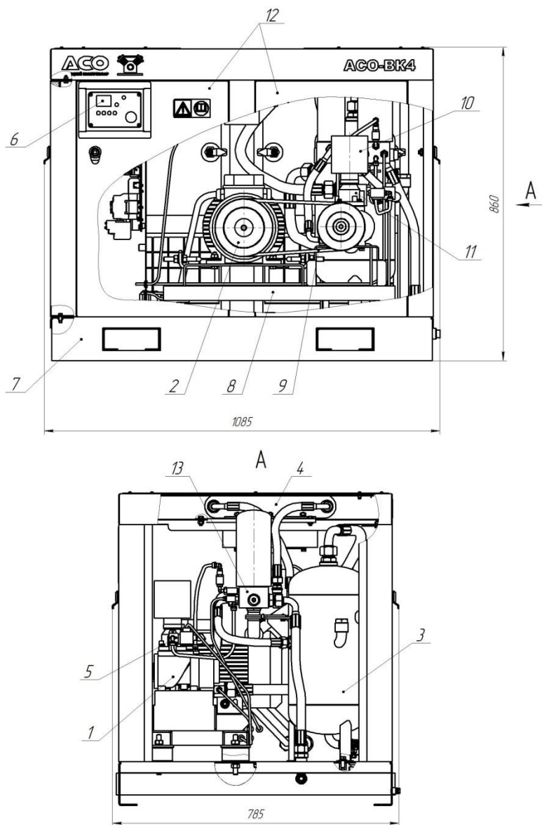
Рисунок 2. Агрегат компрессорный.
